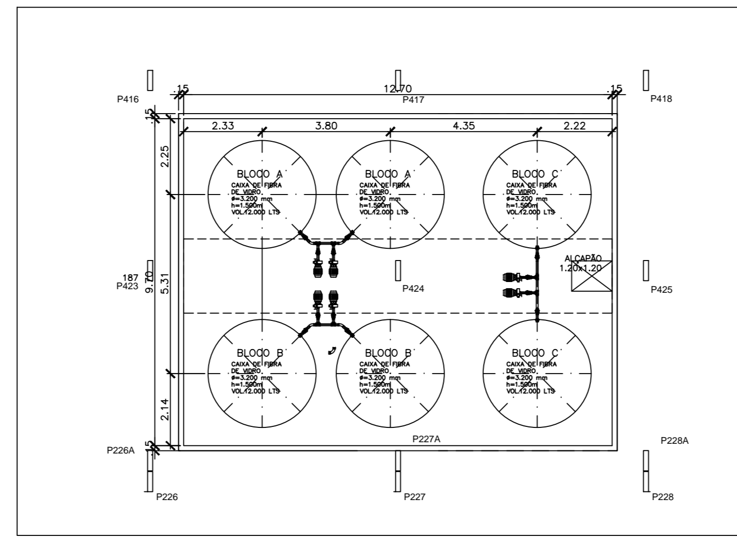
ESTUDO-2 DE ESPAÇO PARA CAIXAS D'AGUA INFERIORES COM CAPACIDADE PARA 12.000 LITROS, DIÂMETRO DE 3,20m, ALTURA DE 1,50m COM PÉ DIREITO DE 2,00 METROS
