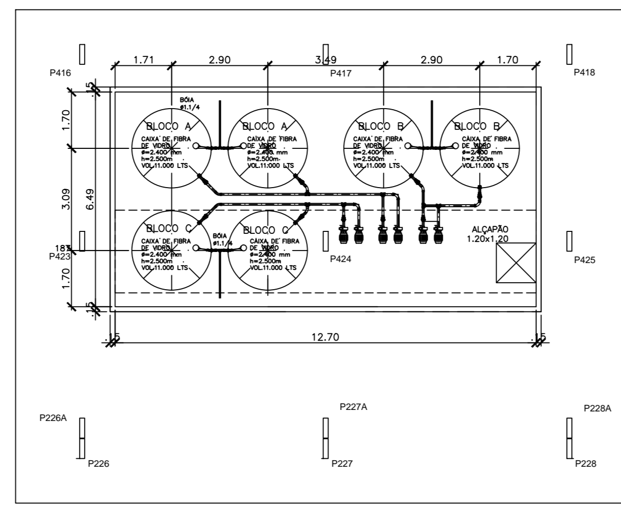
ESTUDO-1 DE ESPAÇO PARA CAIXAS D'AGUA INFERIORES COM CAPACIDADE PARA 11.000 LITROS, DIÂMETRO DE 2,40m, ALTURA DE 2,50m COM PÉ DIREITO DE 3,00 METROS
